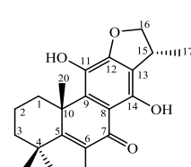
Lycoxanthol (HPB)
